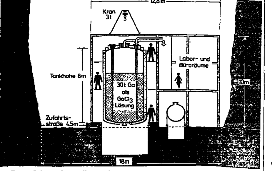
In diesem Jahr beginnen die Arbeiten an dem Gebäude, das in einer Kaverne den 80 000-Liter-Tank für den Gallium-Chlorid-Detektor aufnimmt. SKIZZE: MPG
